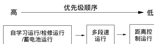
图7-3 控制功能优先级
