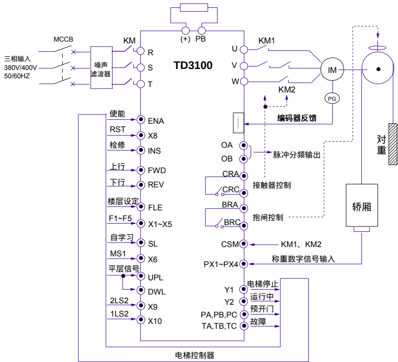
图7-29 控制原理设计示意图（典型应用例二）
