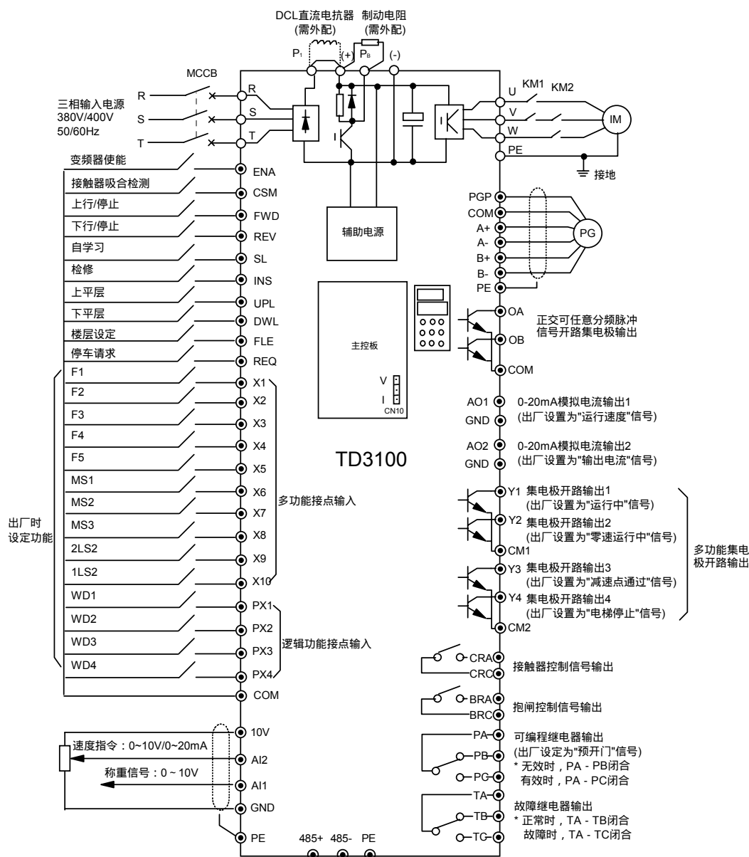
图3-8 基本配线图1
