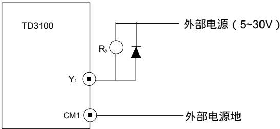
图3-21 开路集电极输出端子接线图2
