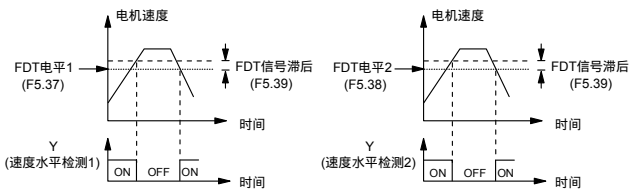
图6-29 速度水平检测示意图
