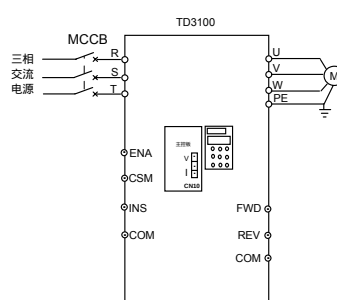
图4-13 试运行配线图1
