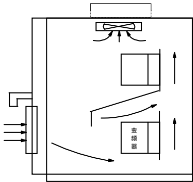
图3-2 多台变频器的安装
