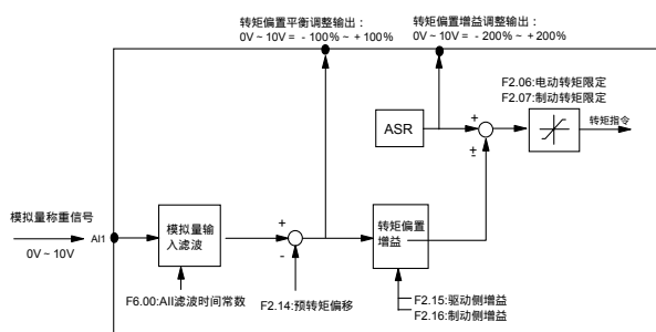
图6-12 转矩偏置调整框图
