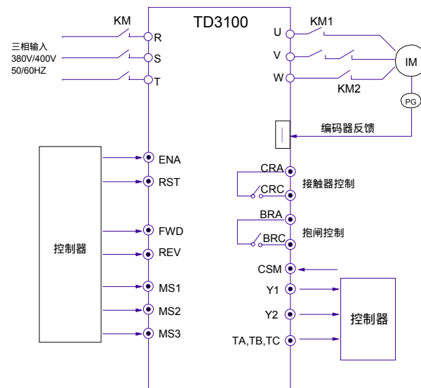
图7-4 多段速度运行基本接线图
