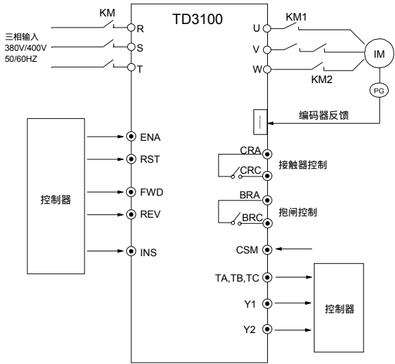
图7-16 检修运行基本接线图
