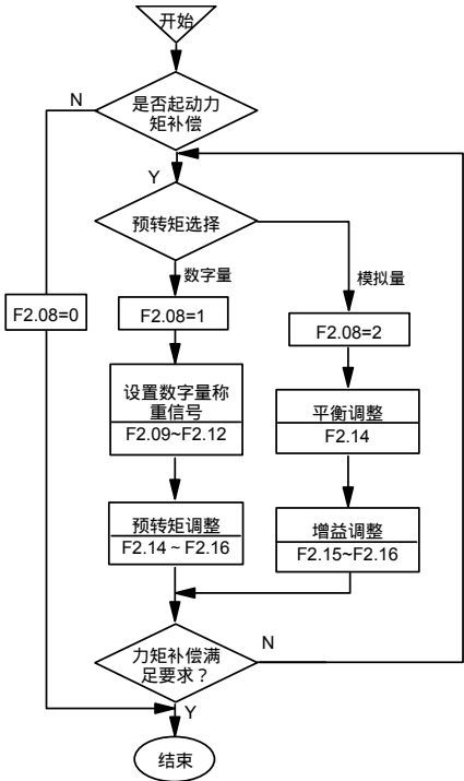
图7-22 启动力矩补偿参数设置步骤
