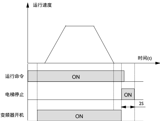
图6-27 运行状态输出示意图
