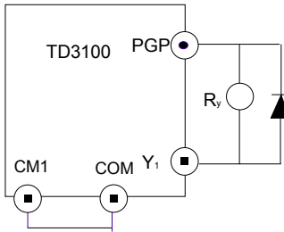
图3-20 开路集电极输出端子接线图1
