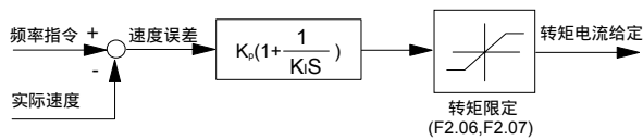
图6-6 速度调节器简化框图
