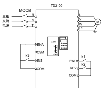
图4-14 试运行配线图2
