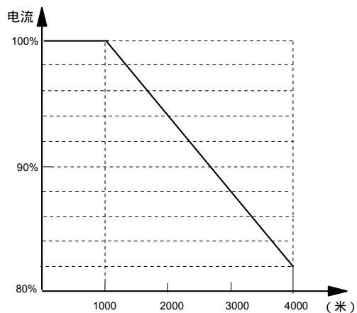
图1-3 变频器额定输出电流与海拔高度关系图
