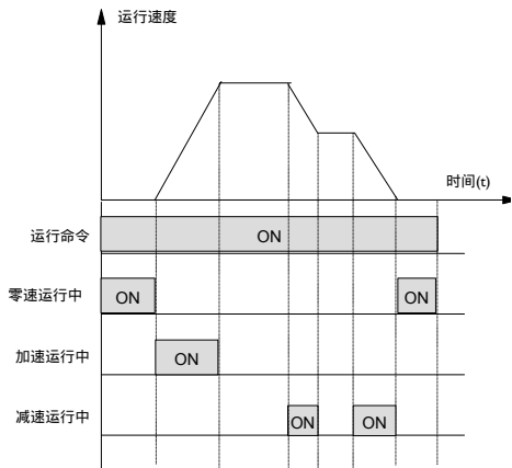
图6-26 运行状态输出示意图
