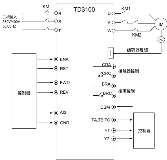
图7-10 普通运行基本接线图
