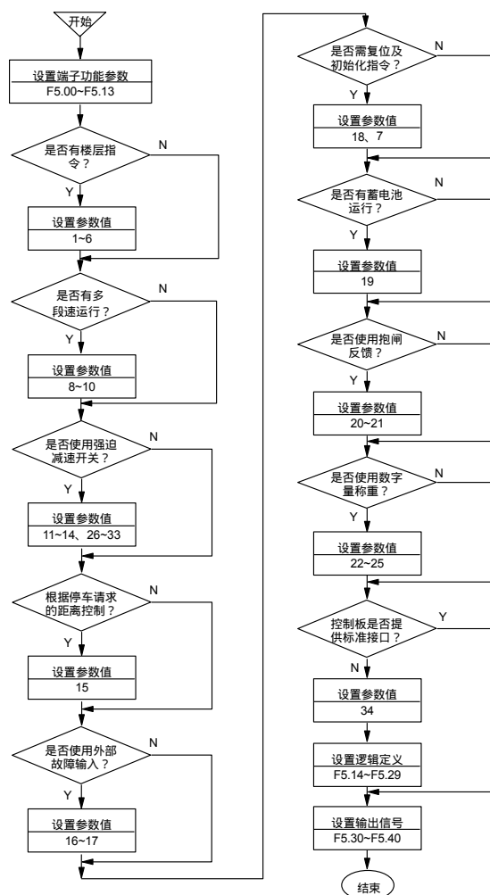
图7-26 可编程端子功能参数设置步骤
