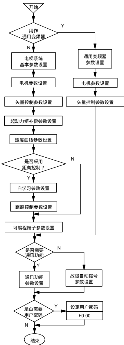
图7-18 电梯应用参数设置总体步骤
