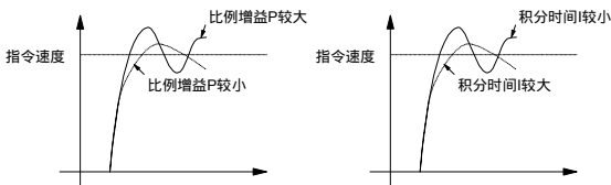
图6-7 速度调节器（ASR）的阶跃响应与PI参数的关系
