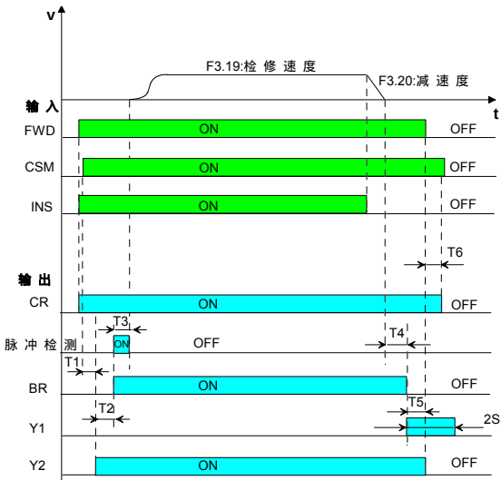
图7-17 检修运行时序
