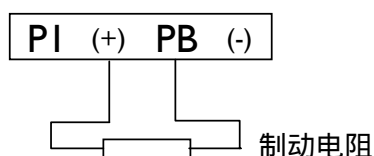
图3-15 制动电阻安装图
