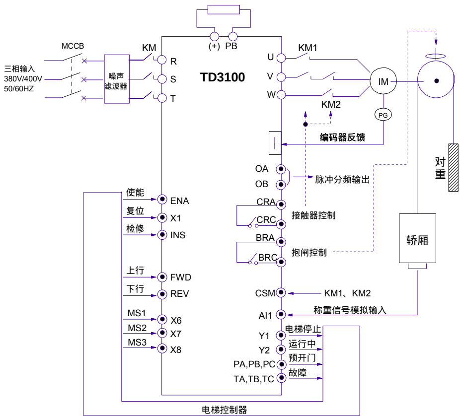
图7-28 控制原理设计示意图（典型应用例一）
