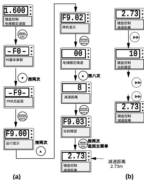
图4-9 停机切换参数流程图
