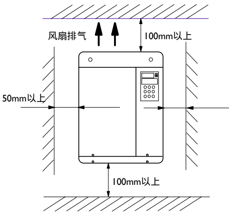
图3-1 安装的间隔距离
