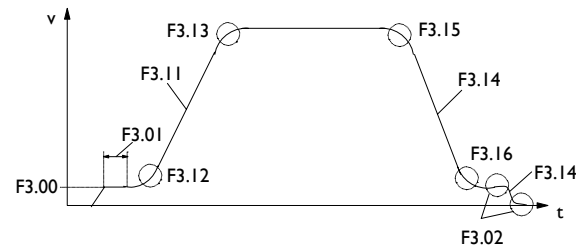
图6-16 S曲线参数示意图
