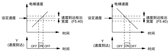
图6-30 速度到达检出示意图
