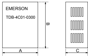
图10-2 制动单元外形尺寸示意图
