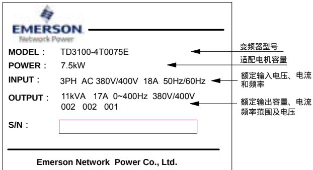
图1-1 变频器铭牌
