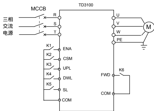
图6-18 自学习运行接线图
