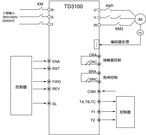
图7-12 自学习运行基本接线图
