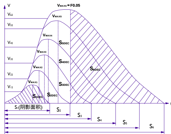
图6-22 距离控制运行的曲线
