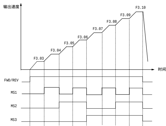
图6-15 多段速度运行示意图
