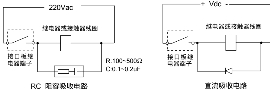
图3-22 浪涌电压吸收电路
