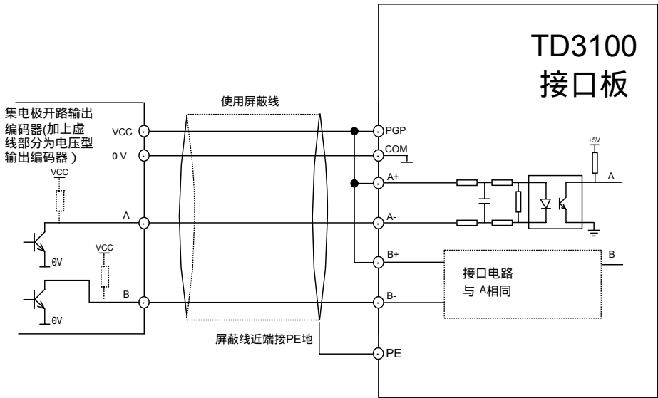
图3-24 集电极开路信号PG接线示意图
