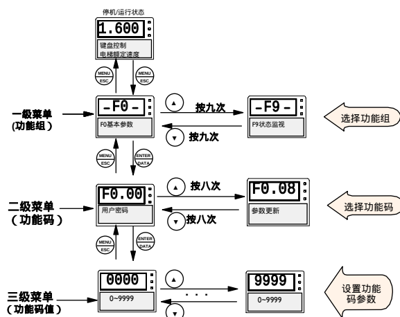
图4-7 三级菜单流程图
