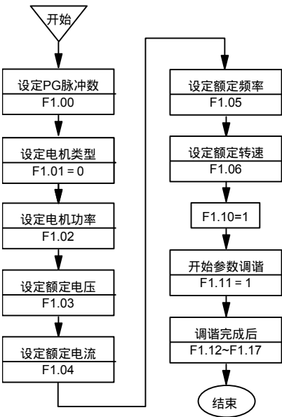
图7-21 电机参数设置步骤
