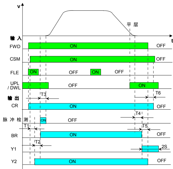
图7-7 给定目的楼层的距离控制运行时序图
