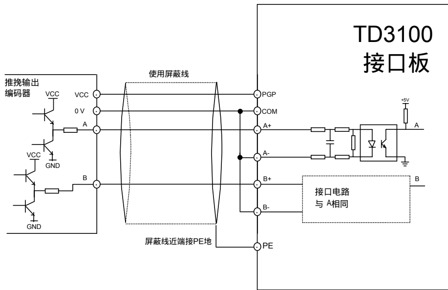
图3-25 推挽信号PG接线示意图
