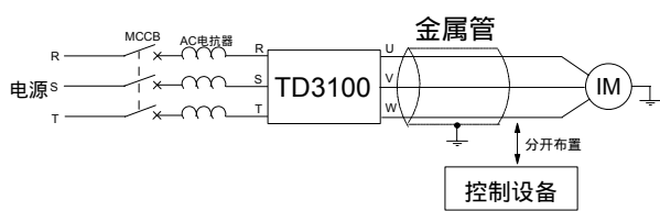
图3-12 变频器输出侧滤波器安装图
