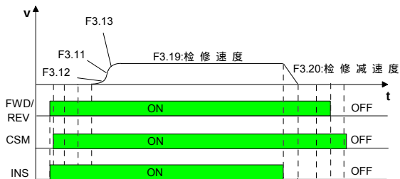
图6-21 检修运行曲线图
