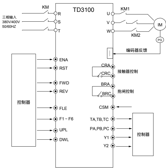
图7-6 给定目的楼层的距离控制运行基本接线图
