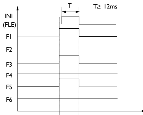
图6-24 INI, FLE指令时序图
