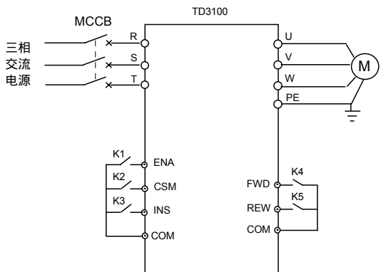
图6-20 检修运行接线图
