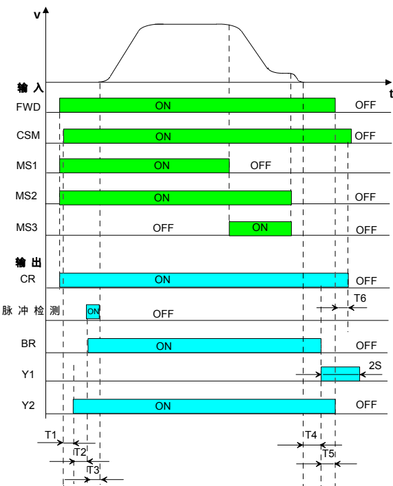
图7-5 多段速度运行时序图
