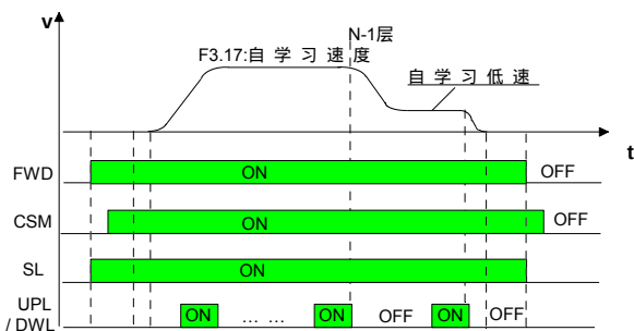
图6-19 自学习运行曲线图
