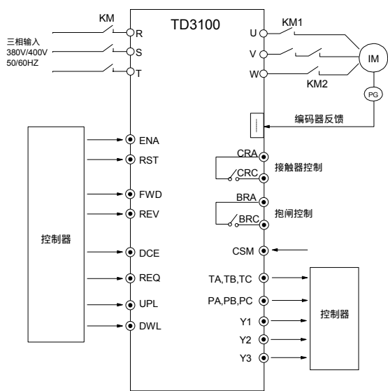
图7-8 给定停车请求的距离控制运行基本接线图
