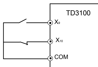
图6-25 上强迫减速常开/常闭输入示意图
