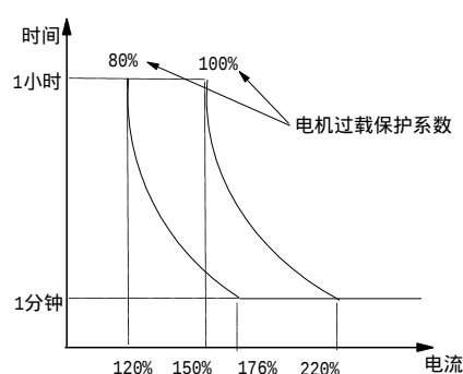
图 6-4 电机过载保护系数设定
