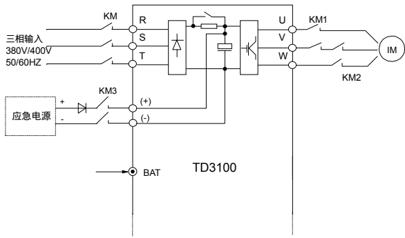
图7-14 蓄电池运行基本接线图
