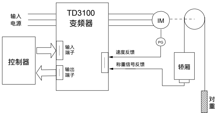
图7-2 典型电梯系统配置图
