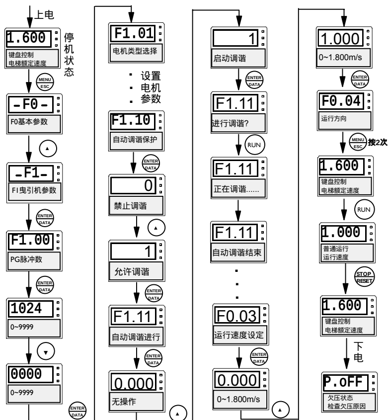
图4-15 详细操作步骤
