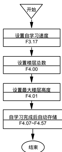
图7-24 自学习参数设置步骤
