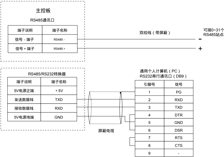
图3-18 串行通讯接口及应用
