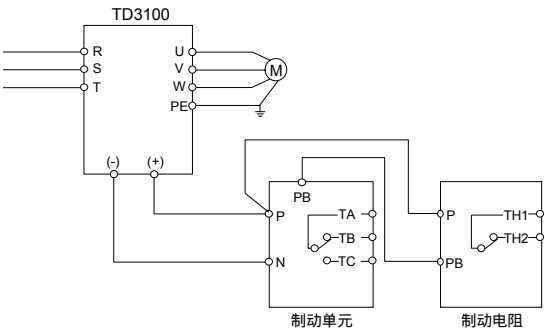
图10-4 变频器与制动阻件连线图
