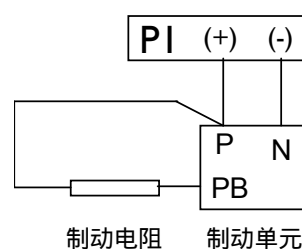
图3-16 制动单元与制动电阻安装图
