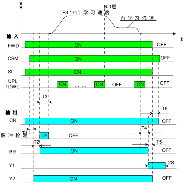
图7-13 自学习运行时序图
