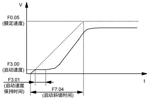
图6-13 启动参数示意图
