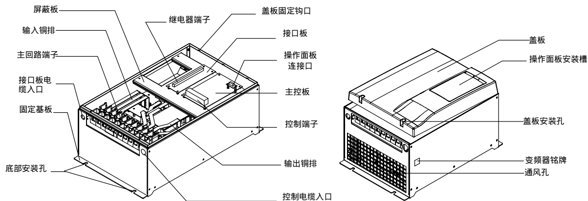
图3-4 18.5kW及以上变频器部件名称
