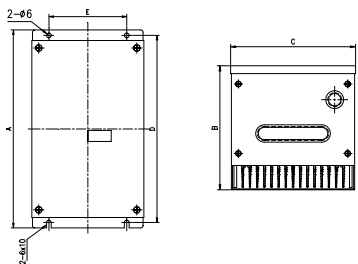
图10-3 制动单元的安装尺寸示意图
