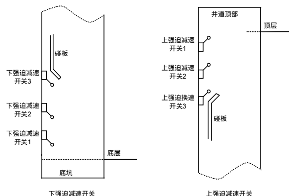
图6-32 三个强迫减速开关示意图
