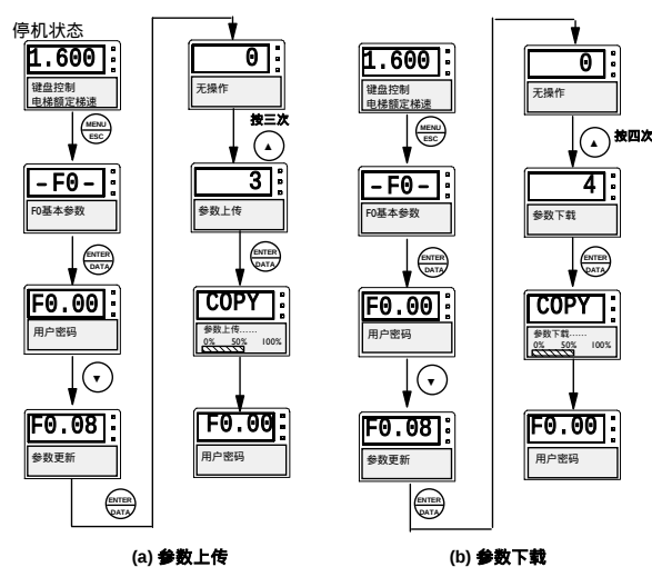
图4-10 参数复制操作流程图
