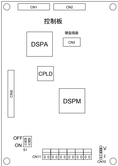
图3-23 控制板跳线位置示意图
