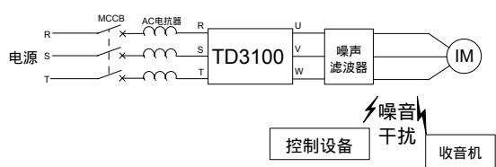
图3-11 变频器输出侧滤波器安装图
