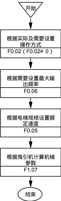
图7-19 电梯基本参数设置步骤
