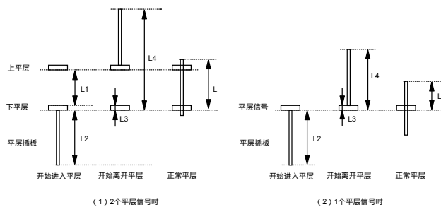
图6-23 距离运行曲线图
