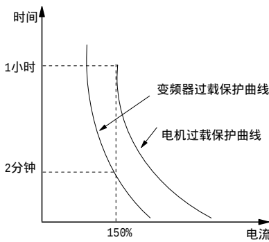
图6-3 变频器过载保护与电机过载保护关系
