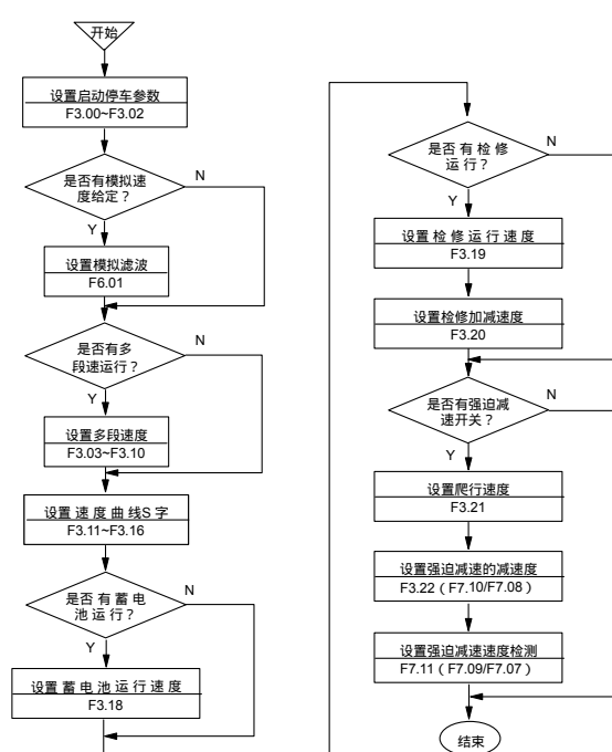
图7-23 速度曲线参数设置步骤
