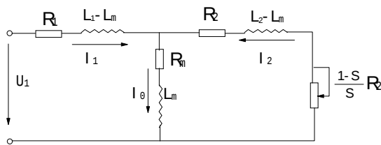
图6-5 异步电机稳态等值电路图
