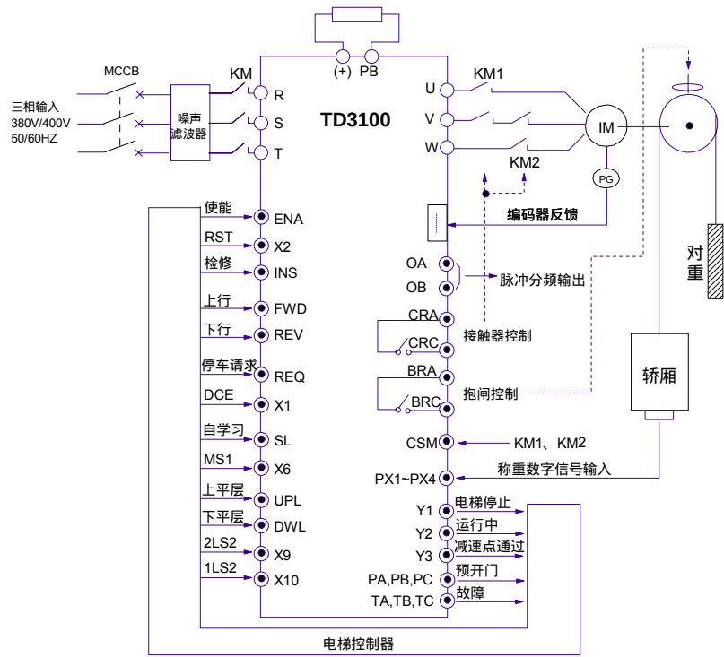
图7-30 控制原理设计示意图（典型应用实例三）
