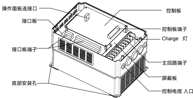
图3-3 18.5kW以下变频器部件名称
