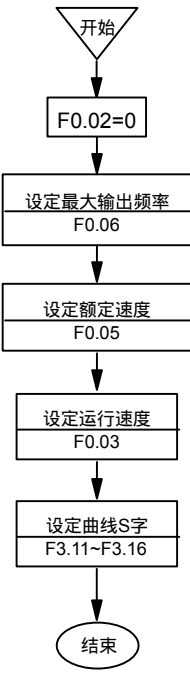
图7-20 通用变频器参数设置步骤
