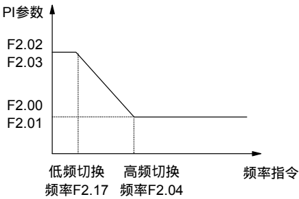
图6-9 PI参数与频率关系示意图
