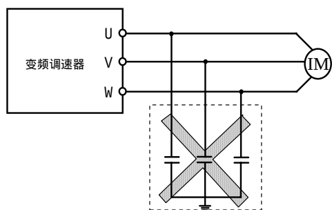
图1-2 变频器输出端禁止使用电容器
