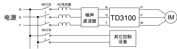
图3-10 电源侧输入滤波器安装图
