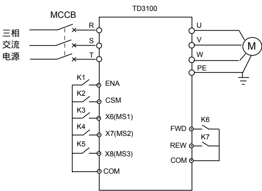
图6-14 多段速度运行接线图
