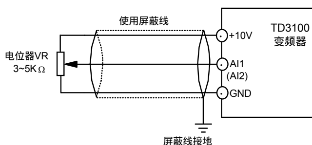
图3-17 模拟输入端子连接
