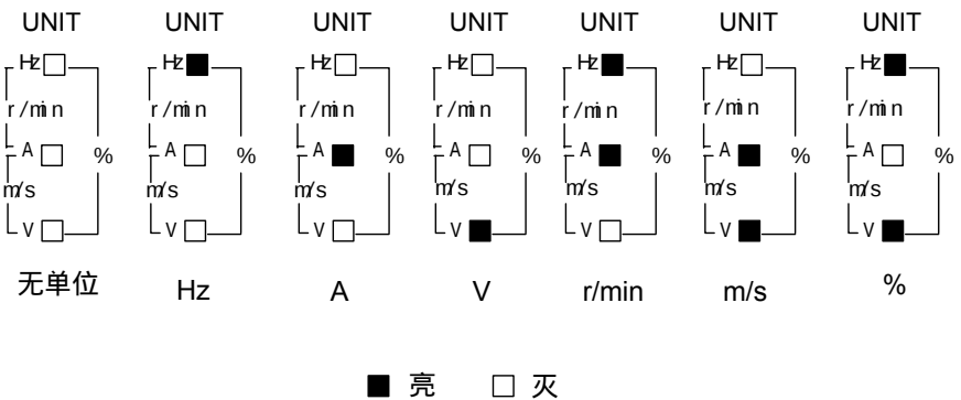
图4-2 单位指示灯状态与单位对应关系图
