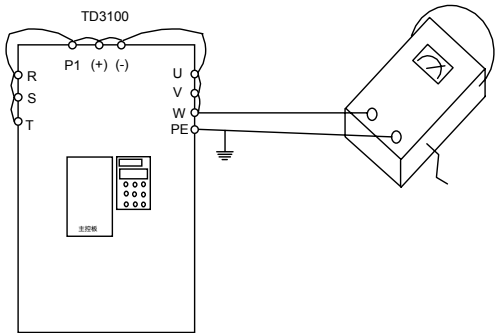
图9-1 变频器绝缘测试图
