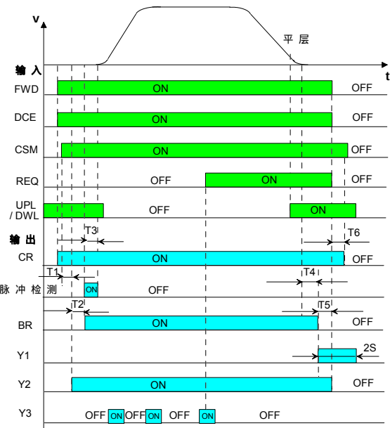
图7-9 给定停车请求的距离控制运行时序图
