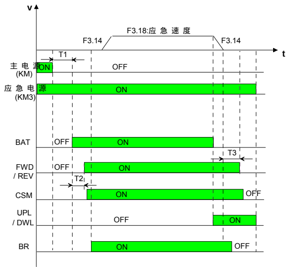
图7-15 蓄电池运行时序图
