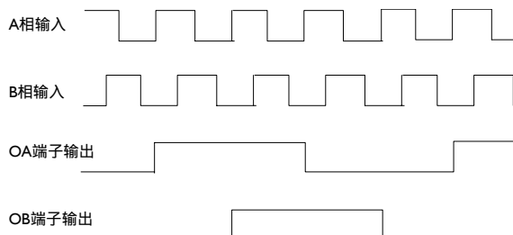
图6-31 4分频波形示意图
