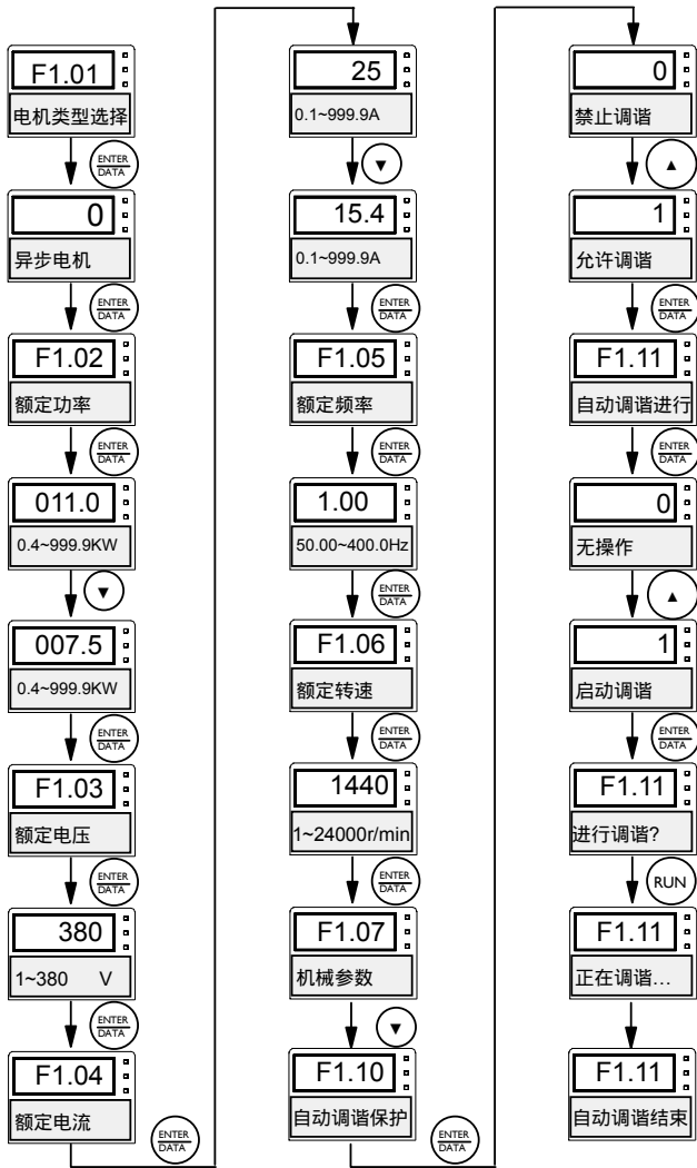
图4-12 参数调谐操作流程
