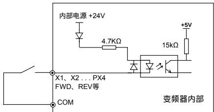
图3-19 使用变频器内部24V电源接点端子连线
