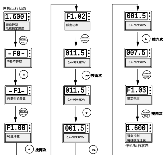
图4-8 设置参数流程图
