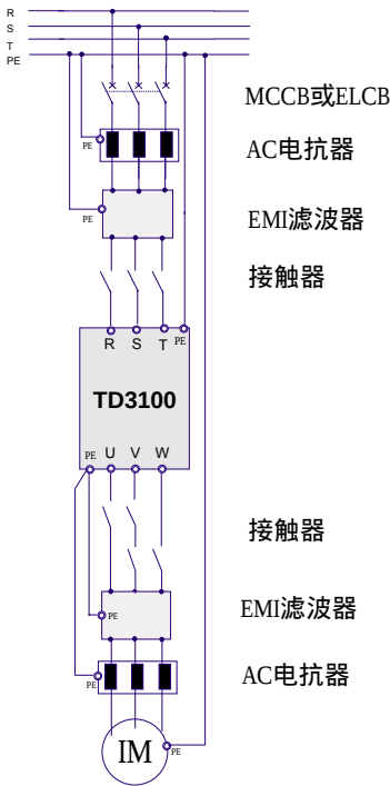
图3-7 外部设备配线图
